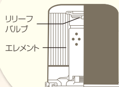
オイルフィルターの構成
